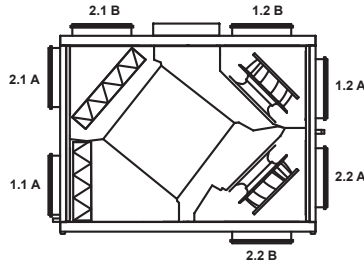
VEX100 - Horizontal/Ceiling RECHTS
