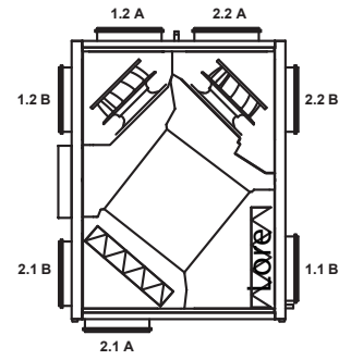
VEX100 - Vertikal RECHTS
