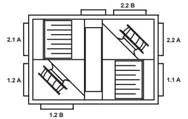
VEX200 - Taschenfilter Ventilatoranordnung 1 - RECHTS
