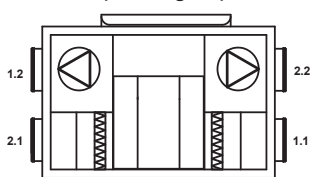
VEX320/330 RECHTS * (Deckengerät)
