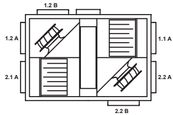
VEX200 - Taschenfilter Ventilatoranordnung 1 - LINKS
