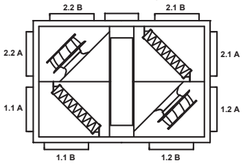
VEX200 - Kompaktfilter Ventilatoranordnung 1 - LINKS
